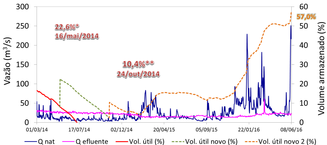
Figura 3. Evolução da vazão afluente (Qnat) do Sistema Cantareira (linha azul), da vazão efluente (Q efluente= vazão para atendimento da demanda Região Metropolitana de São Paulo e Região de Campinas + vazão a jusante (linha magenta), e do volume útil (em porcentagem) do Sistema Cantareira (linha vermelha), do novo volume útil 1 (linha verde, considerando volume útil + volume morto 1*) e do novo volume útil 2 (linha laranja, considerando volume útil + volume morto 1 + volume morto 2**). (Fonte: SABESP – Situação dos mananciais).
