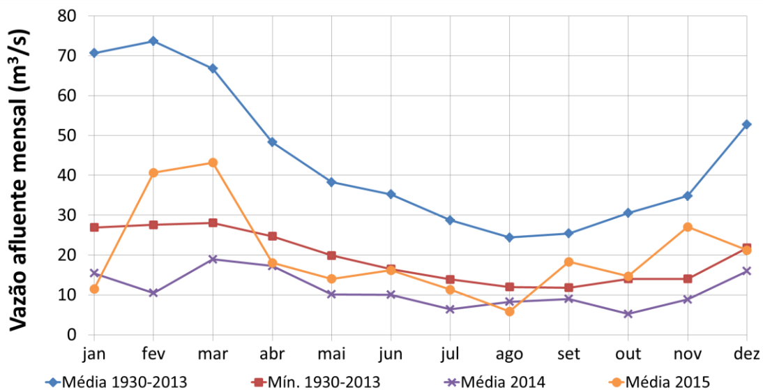
Figura 2. Vazão afluente (em m^3/s ) do Sistema Cantareira (Sistema Equivalente + Paiva Castro). A linha laranja refere-se à vazão média mensal até 02 de dezembro de 2015 e a roxa à vazão média mensal de 2014. As linhas em azul e vermelho correspondem, respectivamente, às vazões médias mensais para o período 1930 – 2013 e aos mínimos absolutos da série histórica mensal no período 1930 – 2013.
