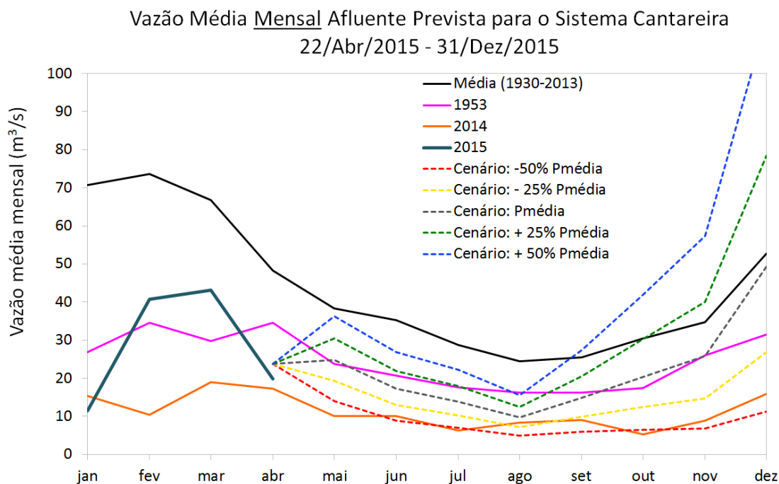
Figura 8. Projeção de vazão média mensal afluyente em m^3/s ao Sistema Cantareira (Sistema Equivalente + Paiva Castro) com a previsão do ETA/CPTEC/INPE para os próximos 7 dias e, na sequência, para 5 cenários: precipitação 50% abaixo da média climatológica (linha vermelha), 25% abaixo da média climatológica (linha amarela), na média climatológica (linha cinza), 25% acima da média climatológica (linha verde) e 50% acima da média climatológica (linha azul). A linha preta refere-se à média mensal climatológica e a laranja aos mínimos absolutos para o período 1930-2013. Em magenta as vazões médias do ano 1953, em roxo de 2014 e em turquesa de 2015, até 22 de abril.
