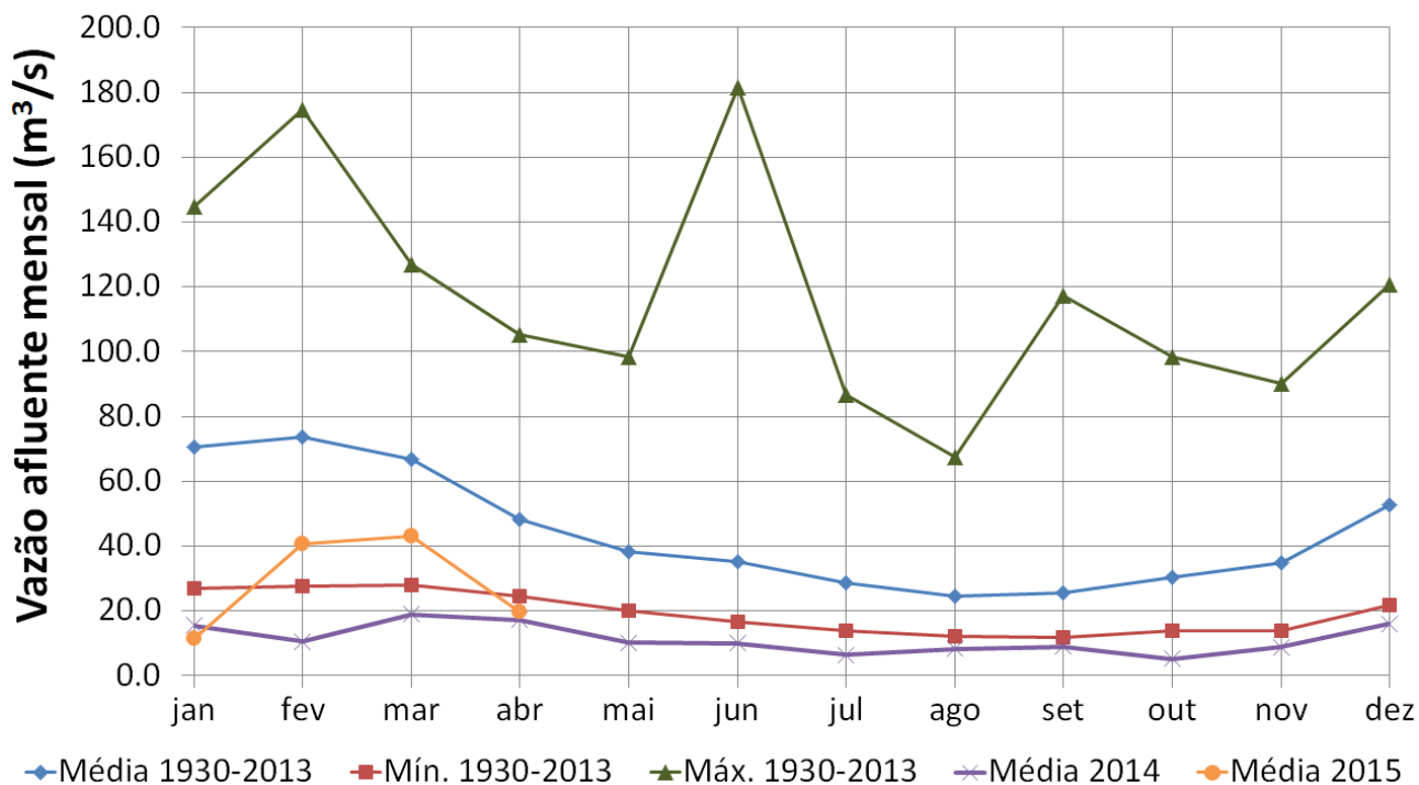
Figura 2. Vazão afluente (em m^3/s ) do Sistema Cantareira (Sistema Equivalente + Paiva Castro). A linha laranja refere-se à vazão média mensal até 22 de abril de 2015 e a roxa à vazão média mensal de 2014. A linha em azul corresponde às vazões médias mensais para o período 1930 – 2013. As linhas verde e vermelha referem-se, respectivamente, aos máximos e mínimos absolutos da série histórica mensal no período 1930 – 2013.
