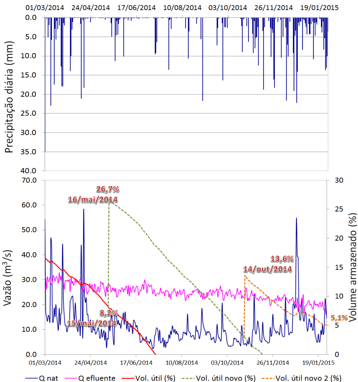
Figura 4. a) Precipitação média diária nas bacias do Sistema Cantareira (Dados do CEMADEN e DAEE) e b) Evolução da vazão afluyente ( Q_{nat} ) do Sistema Cantareira (linha azul), da vazão efluente ( Q_{efluente} = vazão para atendimento da demanda Região Metropolitana de São Paulo e Região de Campinas + vazão a jusante (linha magenta)), e do volume útil (em porcentagem) do Sistema Cantareira (linha vermelha), do novo volume útil 1 (linha verde) e do novo volume útil 2 (linha laranja). As porcentagens correspondem ao volume útil de 981,55 hm 3 (Fonte: SABESP – Situação dos mananciais e boletins diários da ANA – GTAG-Cantareira: situação dos reservatórios).
