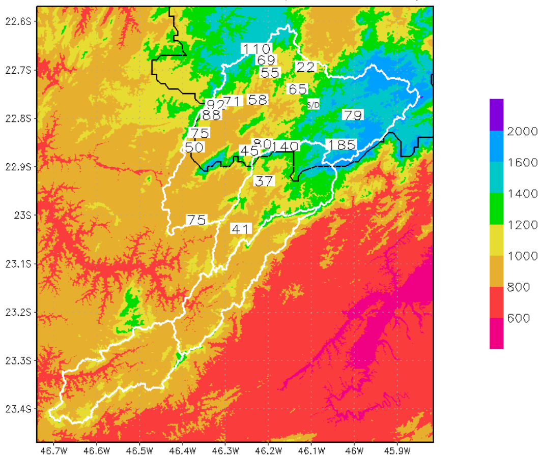
Figura 5. Precipitação observada acumulada do mês, até 28 de janeiro de 2015 (em mm) nos pluviômetros do CEMADEN nas sub-bacias de captação do Sistema Cantareira (contornos em branco). As cores representam alturas topográficas com relação ao nível do mar de acordo com a escala da direita. (s/d) Indica que houve falta de dados em algum período
