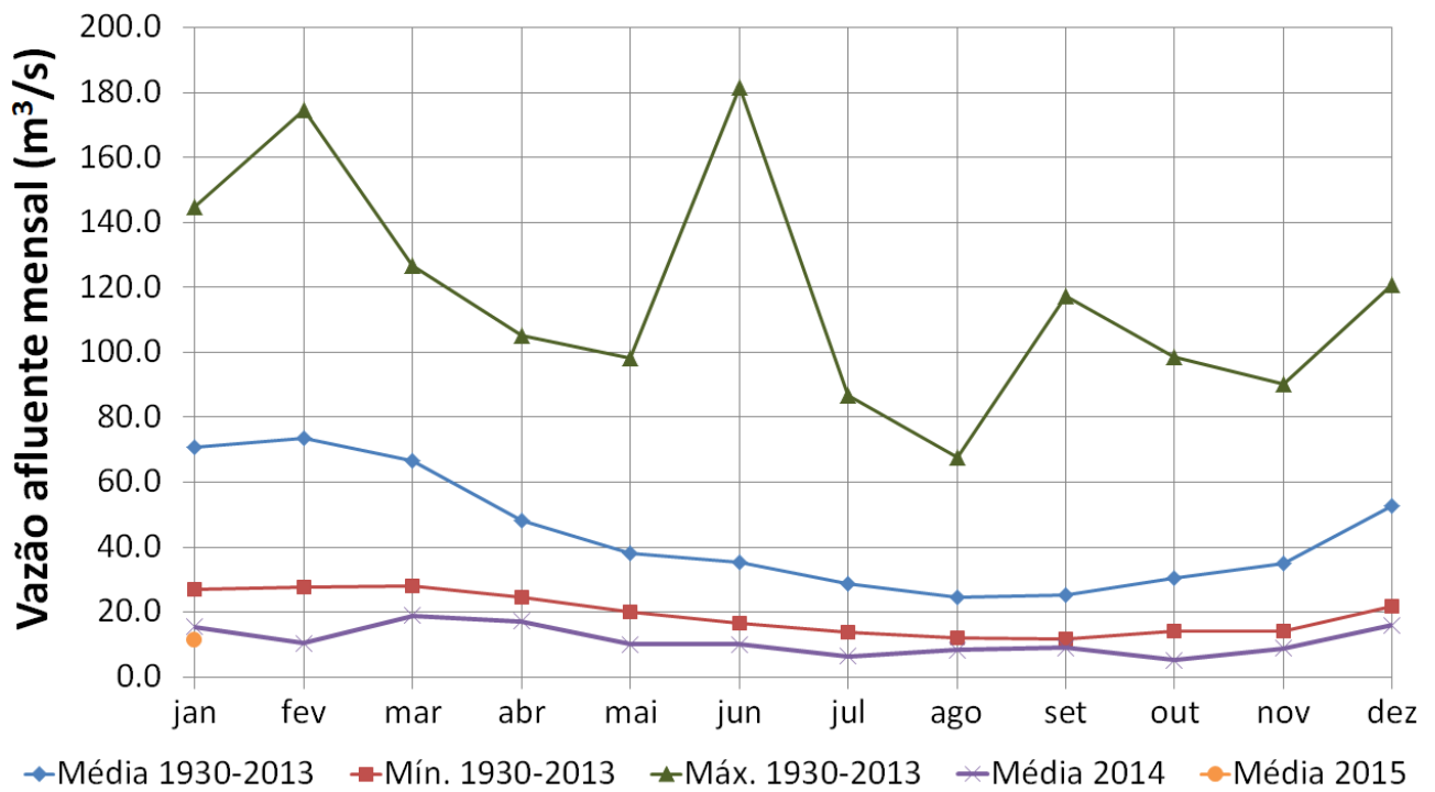
Figura 2. Vazão afluyente (em m^3/s ) do Sistema Cantareira (Sistema Equivalente + Paiva Castro). O ponto em laranja refere-se à vazão média mensal até 29 de janeiro de 2015 e a linha em roxo à vazão média mensal de 2014. A linha em azul corresponde às vazões médias mensais para o período 1930 – 2013. As linhas verde e vermelho referem-se, respectivamente, aos máximos e os mínimos absolutos da série histórica mensal no período 1930 – 2013.
